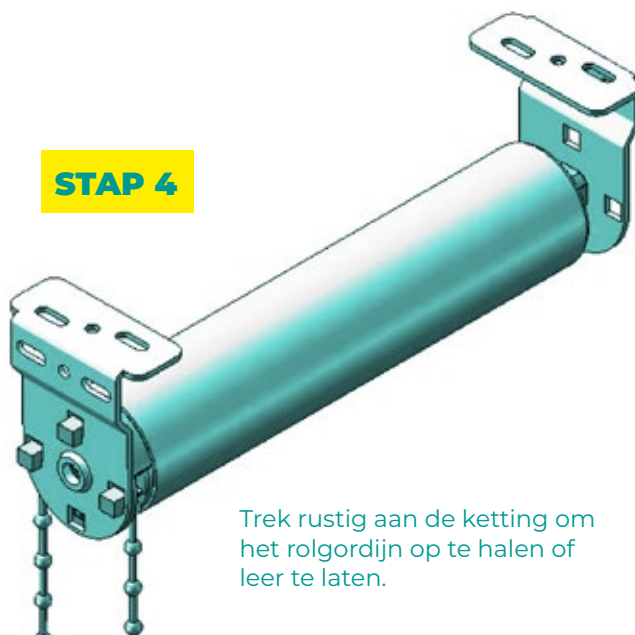
Plafondbevestiging
